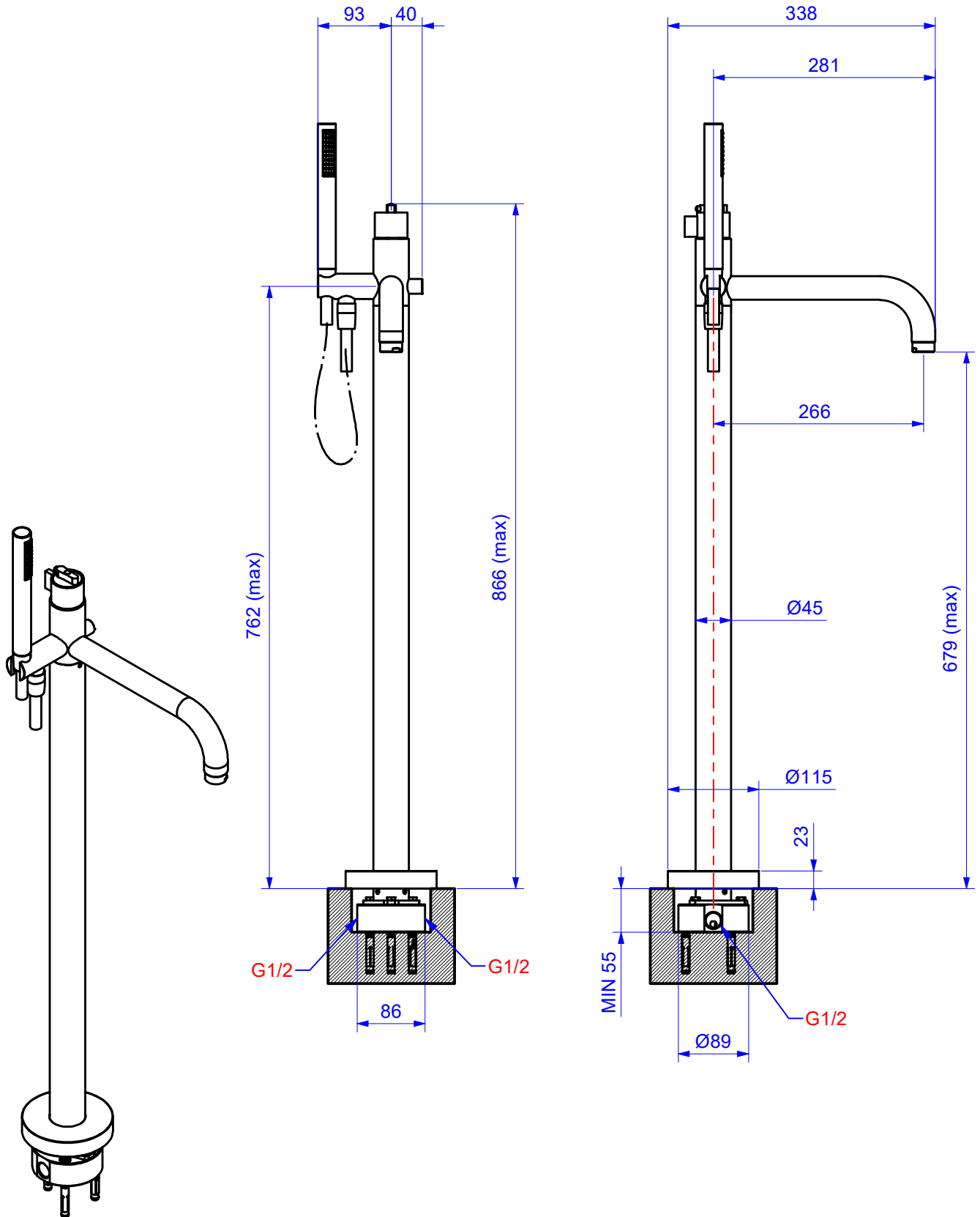
Piantana termostatica a pavimento per riempimento vasca KOBUK
